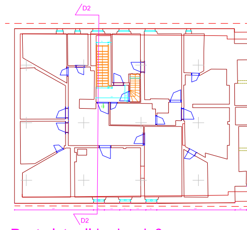
Rzut piętra II budynek 3
